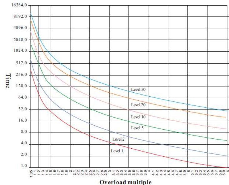
Рисунок 5–6 Кривые характеристик защиты от перегрузки
