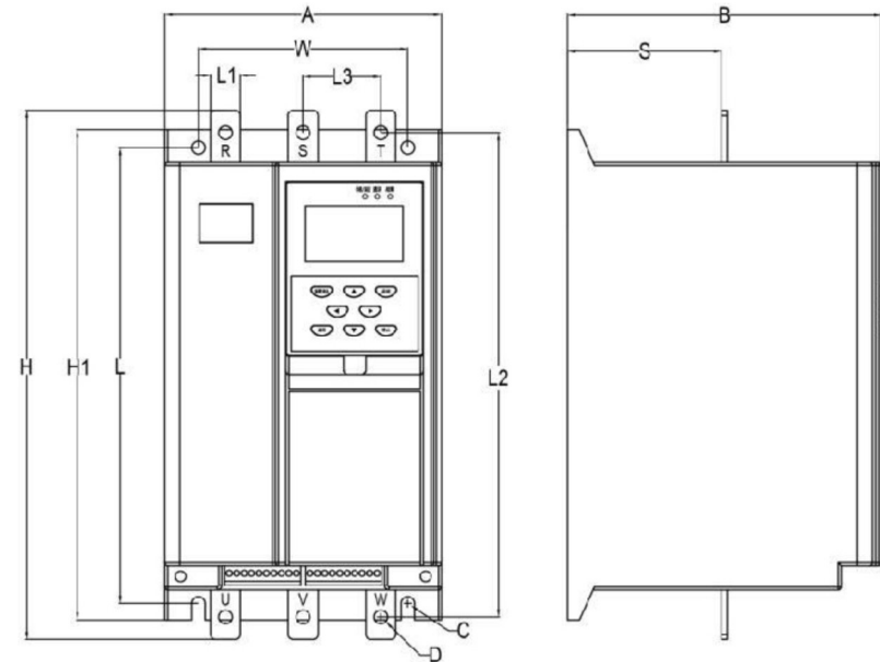
Габаритный чертеж (типоразмер RR1)
