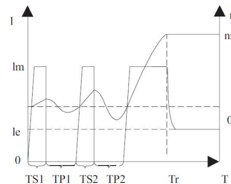
Рисунок 5-5 Пуск с «раскачиванием»
