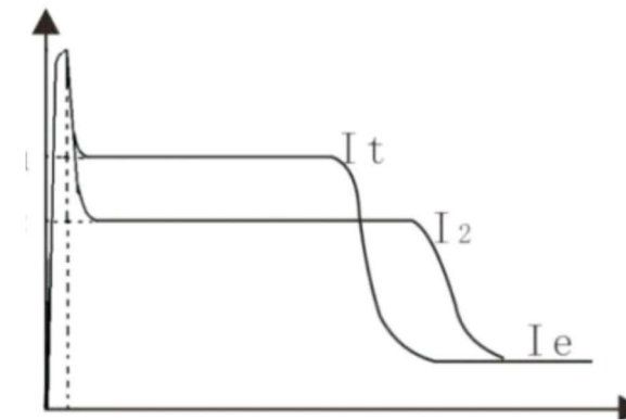
Рисунок 5-3 Пуск со скачком и ограничением тока
