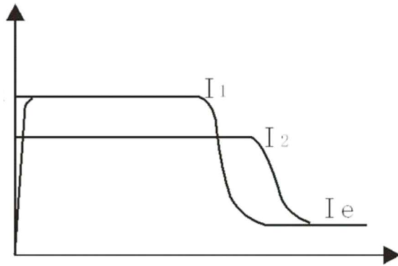
Рисунок 5-1 Пуск с ограничением тока
