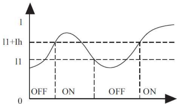
Рисунок 5-8 Работа в режиме «ток выше уставки», тип 2
