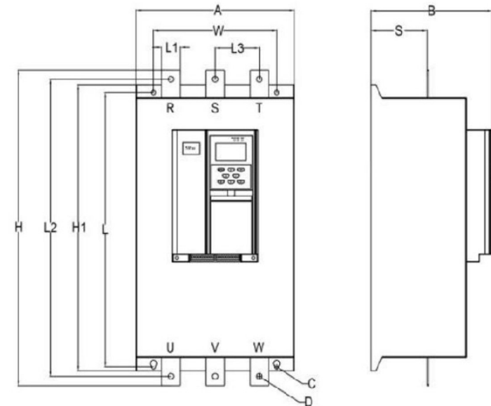
Габаритный чертеж (типоразмер RR2, RR3)
