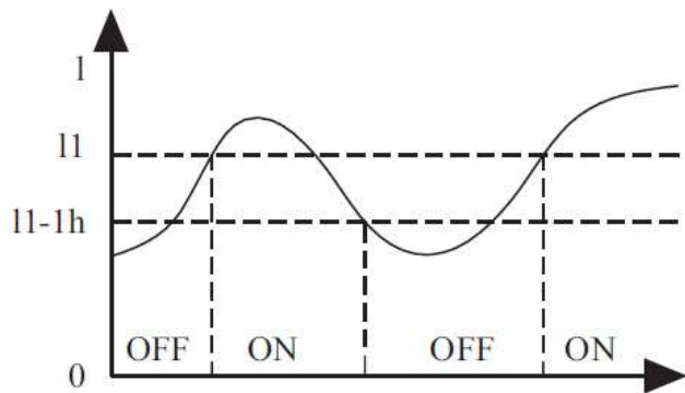
Рисунок 5-7 Работа в режиме «ток выше уставки», тип 1
